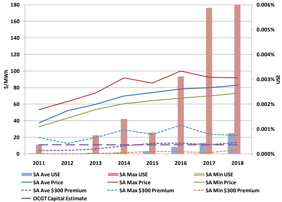
Figure 8-7 SA 50 PoE Projections
