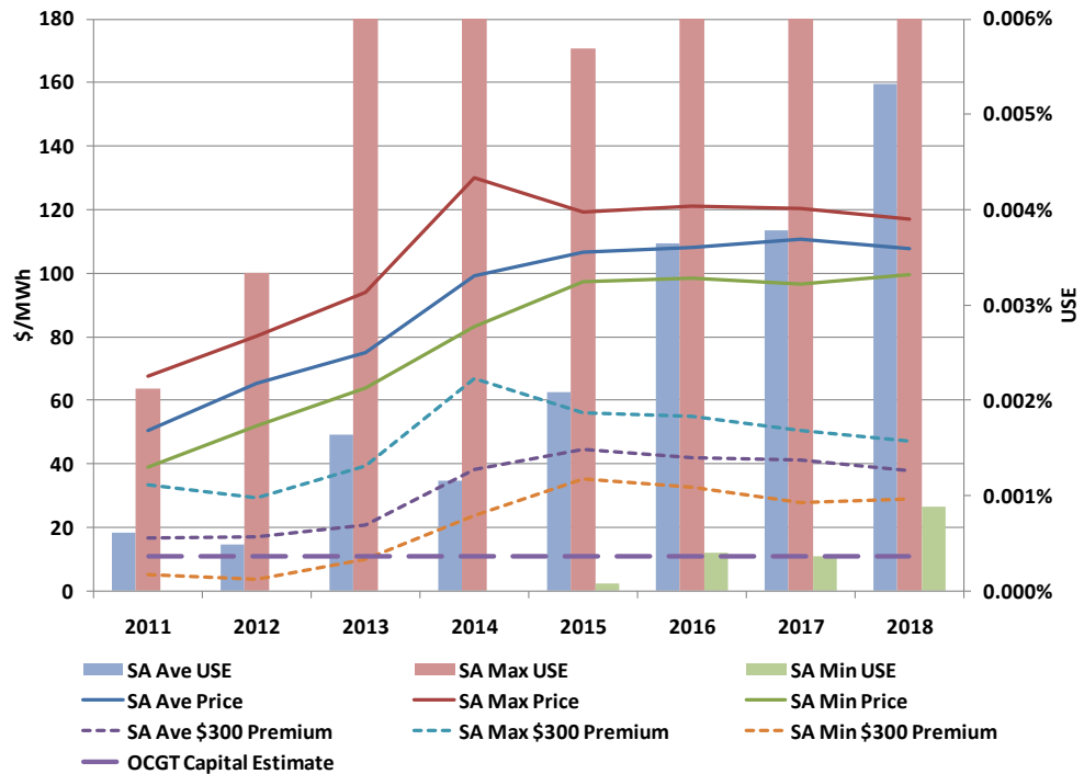
Figure 8-11 SA 10 PoE Projections
