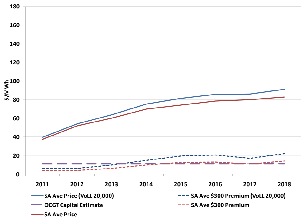
Figure 8-16 SA Comparison
