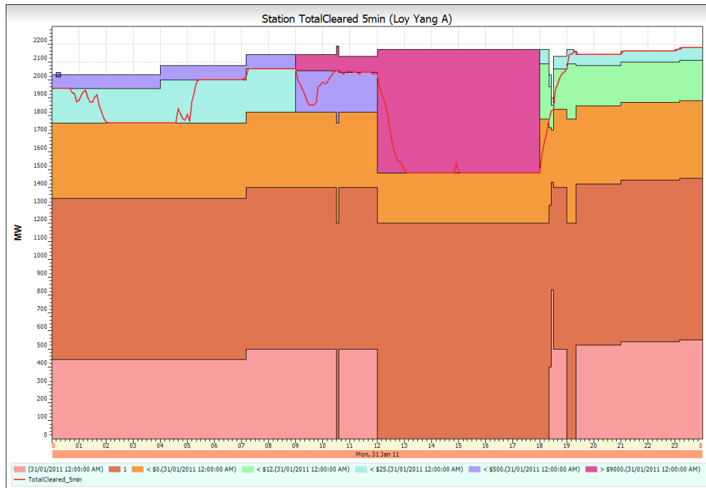
Figure 11-3 Loy Yang A Bids
